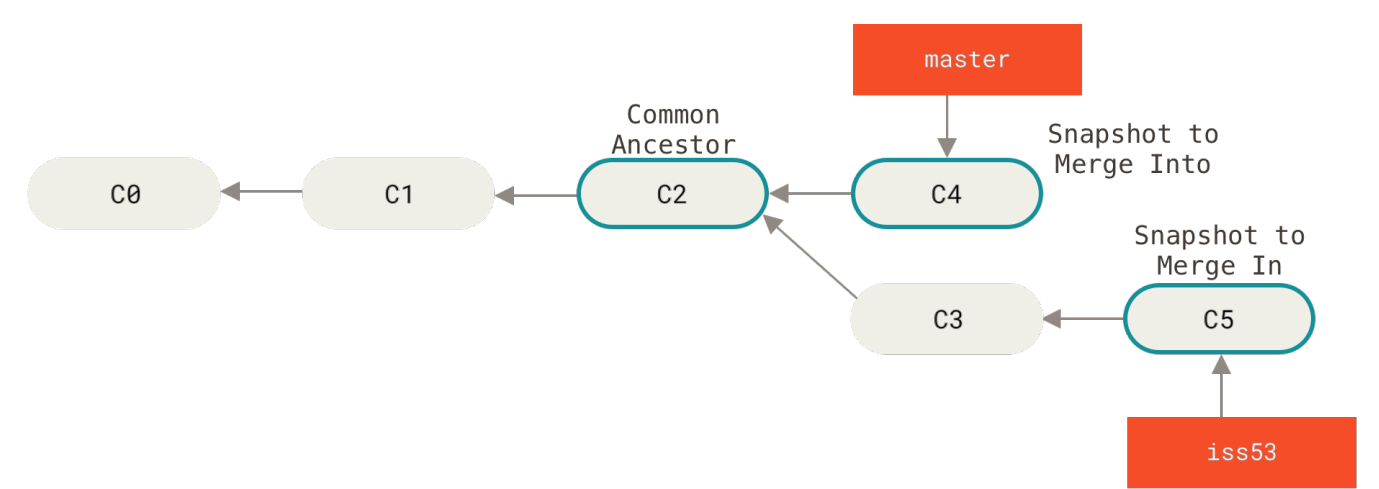
图表 24. 一次典型合并中所用到的三个快照
