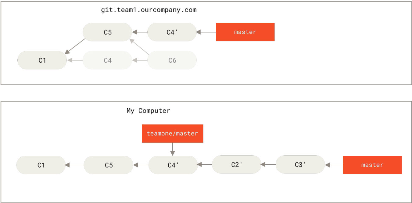
图表 48. 在一个被变基然后强制推送的分支上再次执行变基
