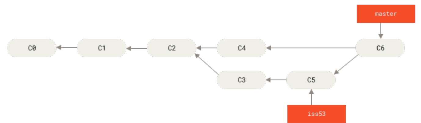
图表 25. 一个合并提交
