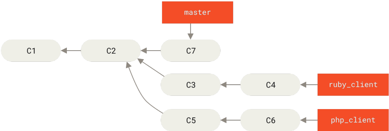
图表 73. 包含若干主题分支的提交历史。
