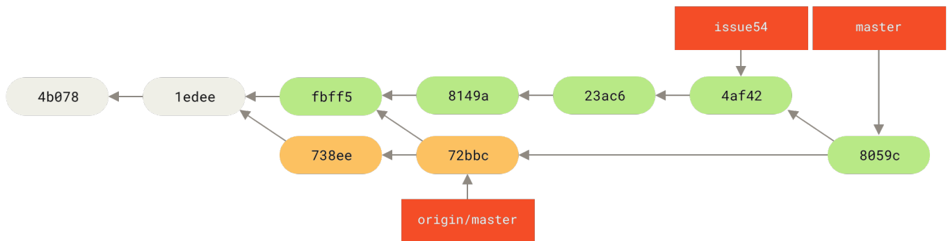
图表 63. 合并了 John 的改动后 Jessica 的历史
