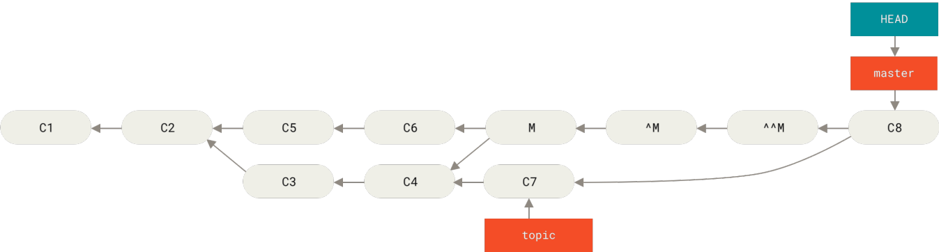
图表 142. 在重新合并一个还原合并后的历史
