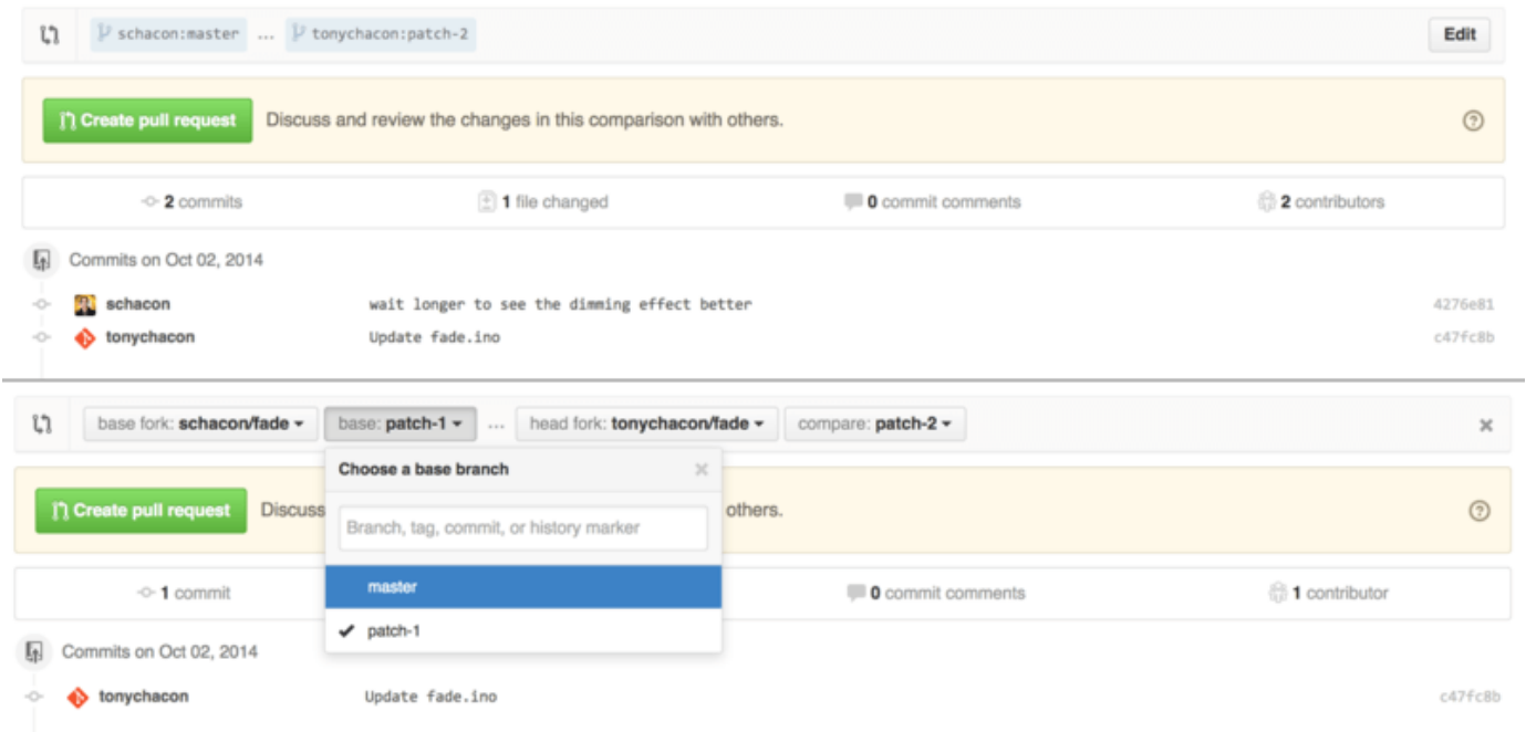
图表 118. 手工修改合并请求的目标。
