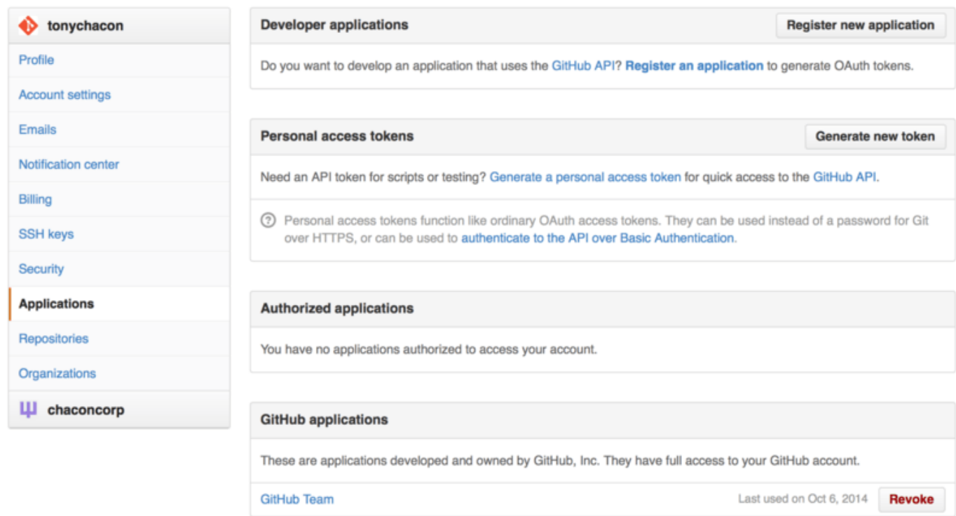
图表 134. 从设置页的“Applications”标签生成访问令牌。
