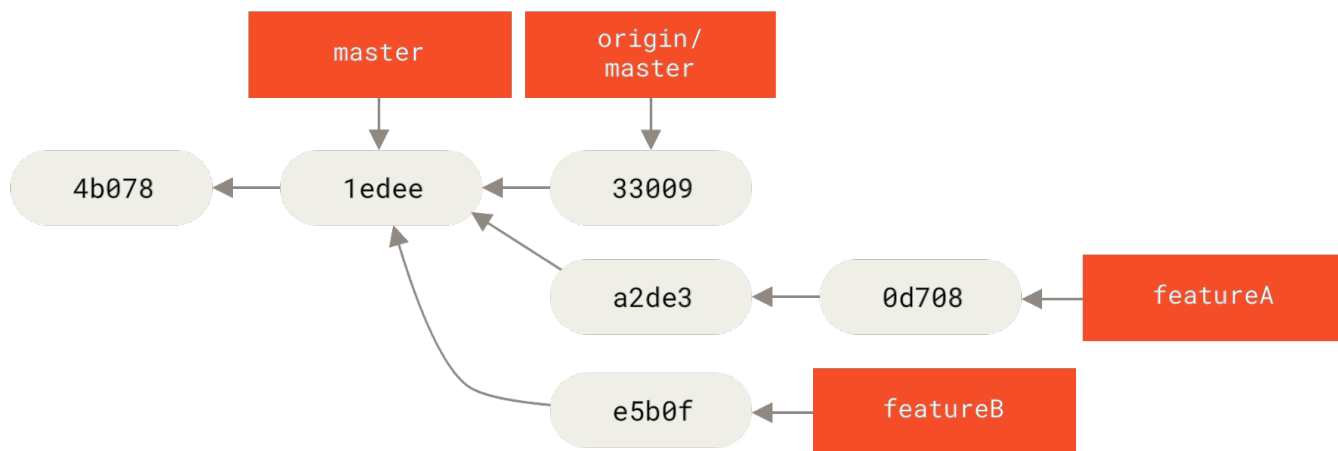
图表 70. featureB 的初始提交历史
