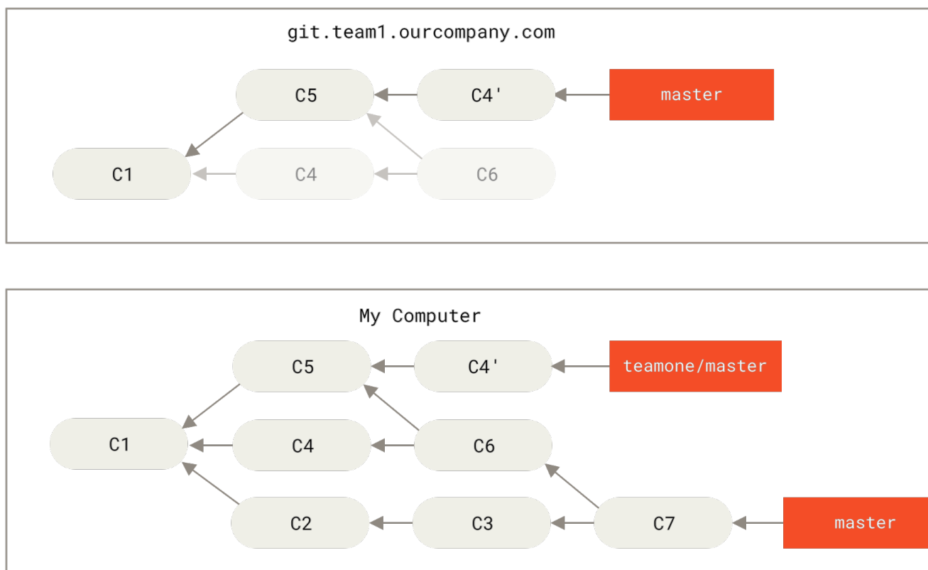
图表 46. 有人推送了经过变基的提交，并丢弃了你的本地开发所基于的一些提交
