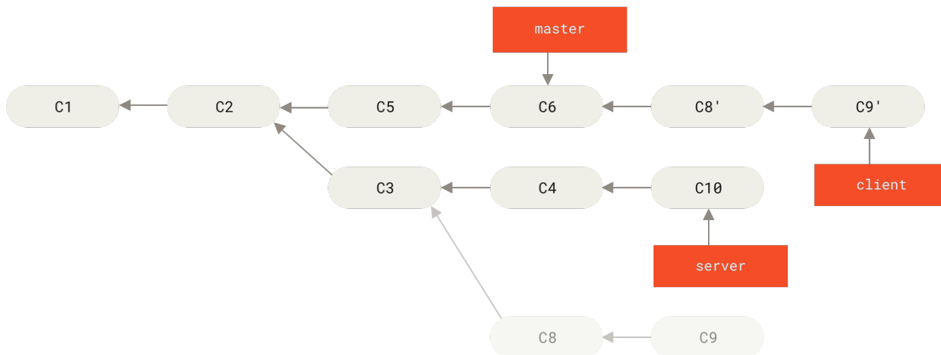
图表 40. 截取主题分支上的另一个主题分支，然后变基到其他分支
