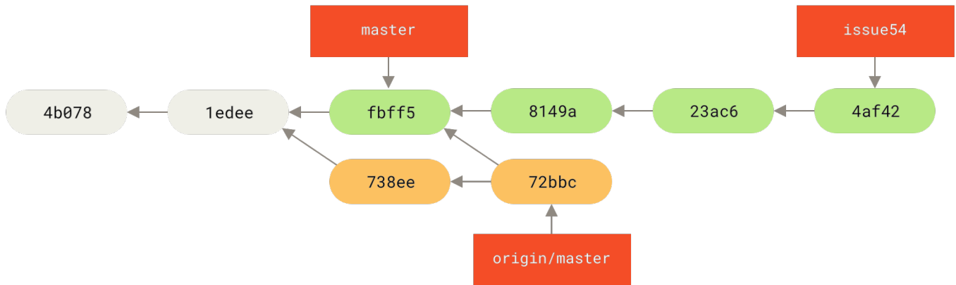
图表 62. 抓取 John 的改动后 Jessica 的历史
