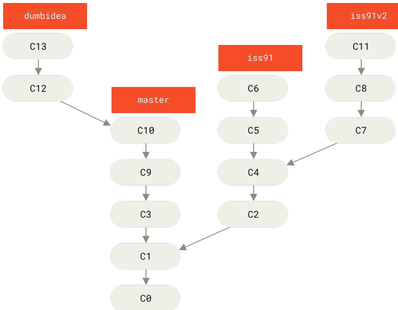
图表 28. 拥有多个主题分支的提交历史
