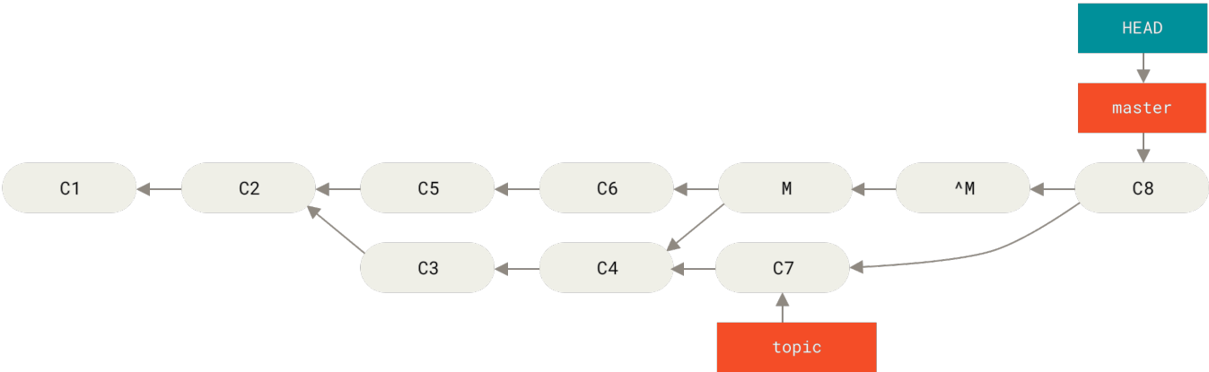
图表 141. 含有坏掉合并的历史
