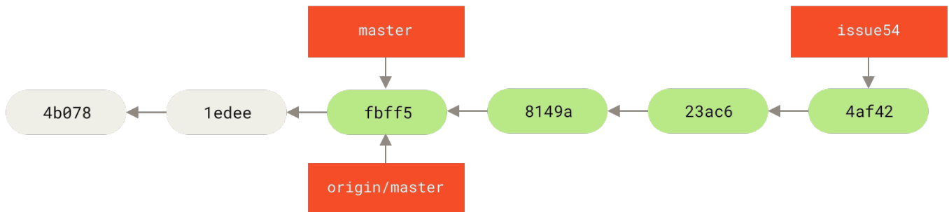
图表 61. Jessica 的主题分支
