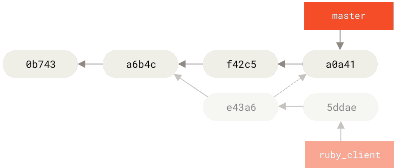
图表 81. 拣选主题分支中的一个提交后的历史。
