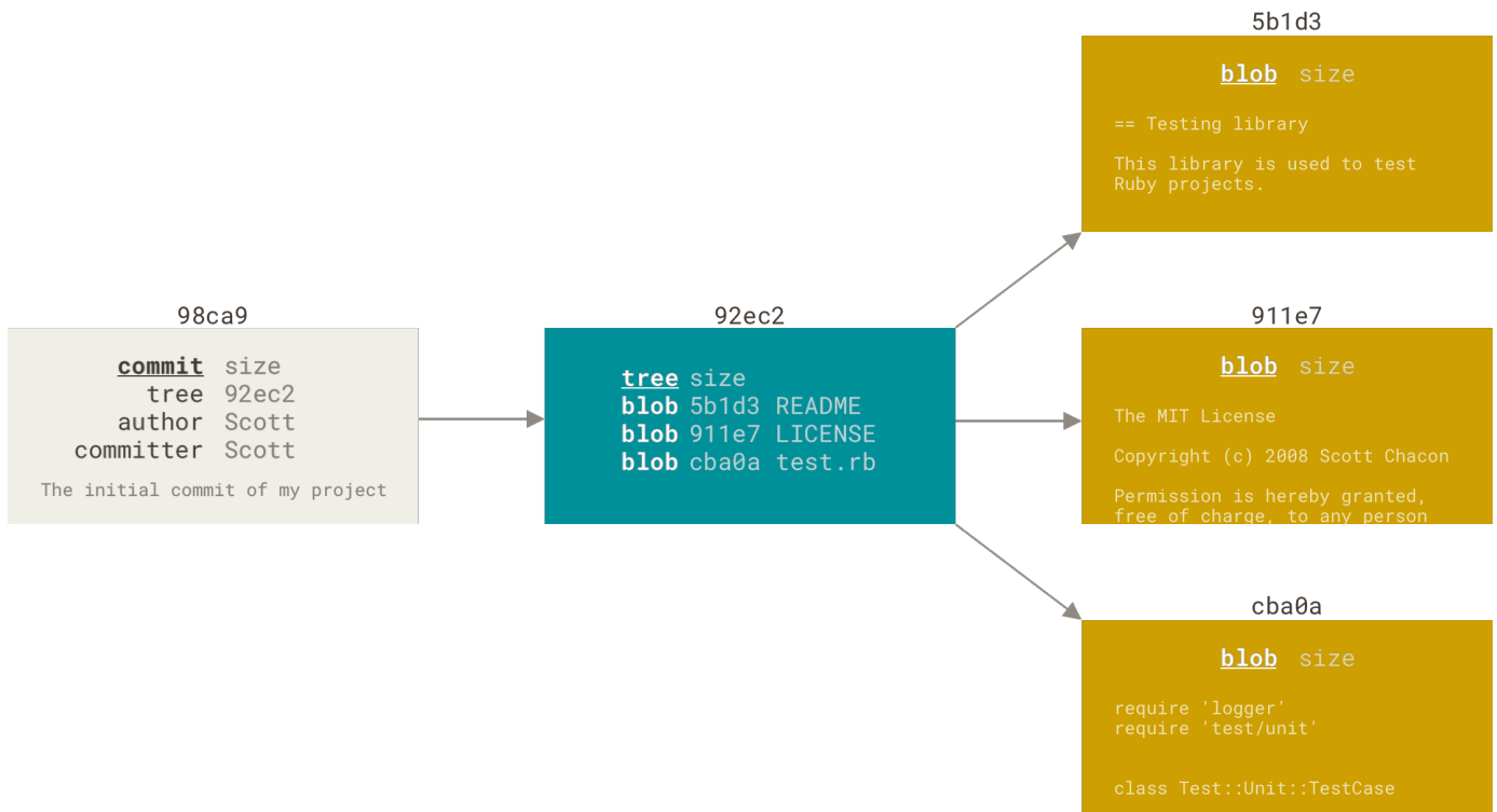
图表 9. 首次提交对象及其树结构
