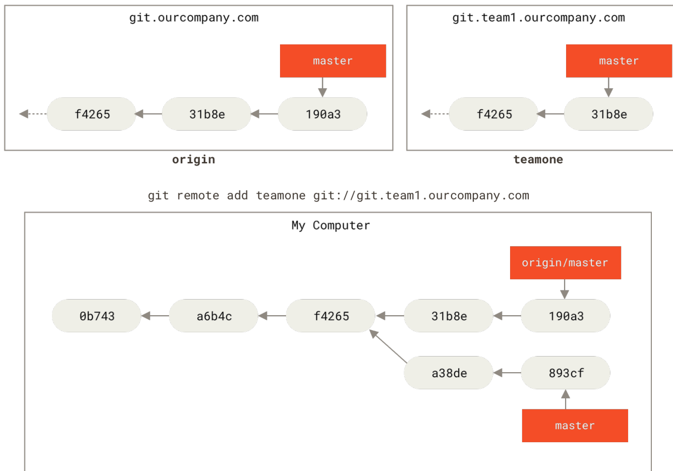
图表 33. 添加另一个远程仓库
