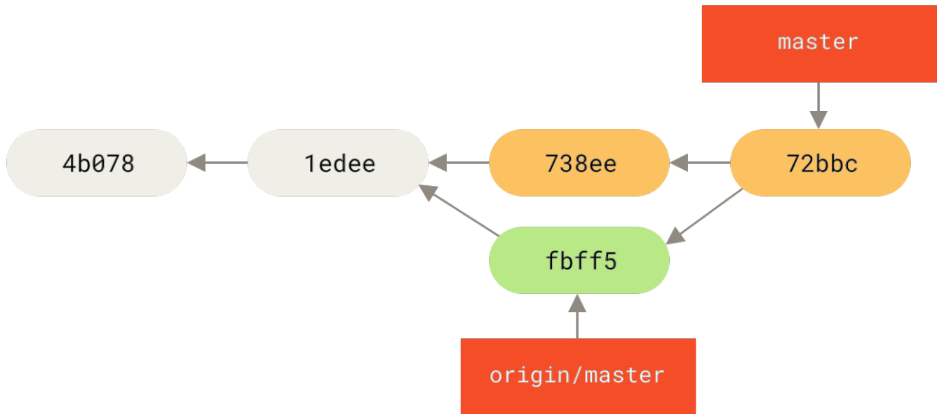
图表 59. 合并了 origin/master 之后 John 的仓库
