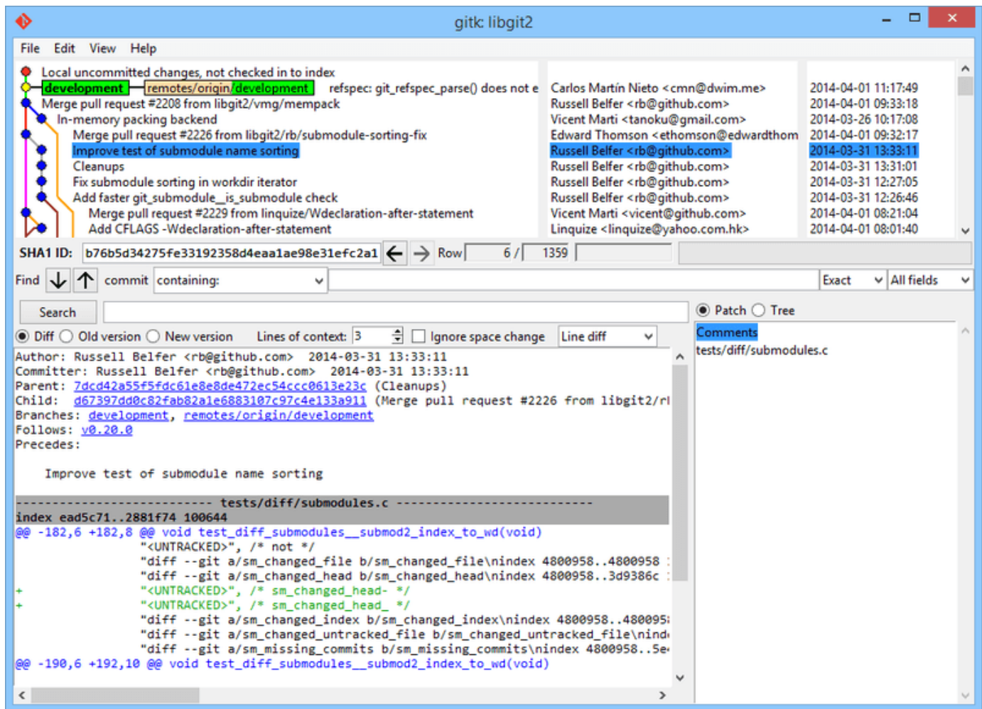
图表 152. gitk 历史查看器。
