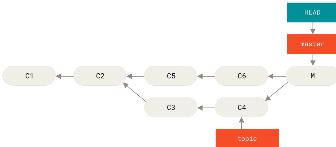
图表 138. 意外的合并提交
