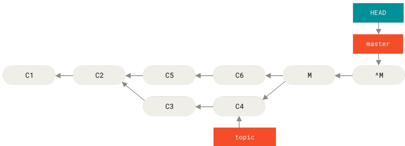
图表 140. 在 git revert -m 1 后的历史
