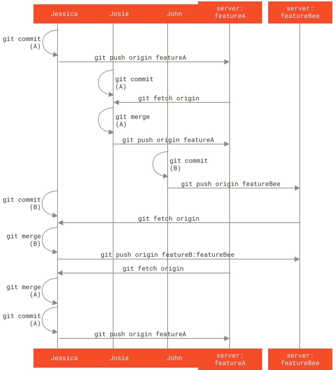
图表 69. 这种管理团队工作流程的基本顺序
