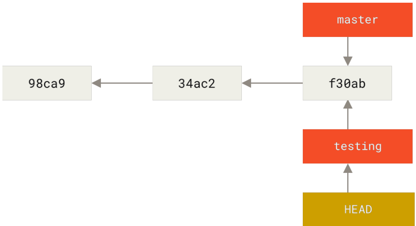
图表 14. HEAD 指向当前所在的分支
