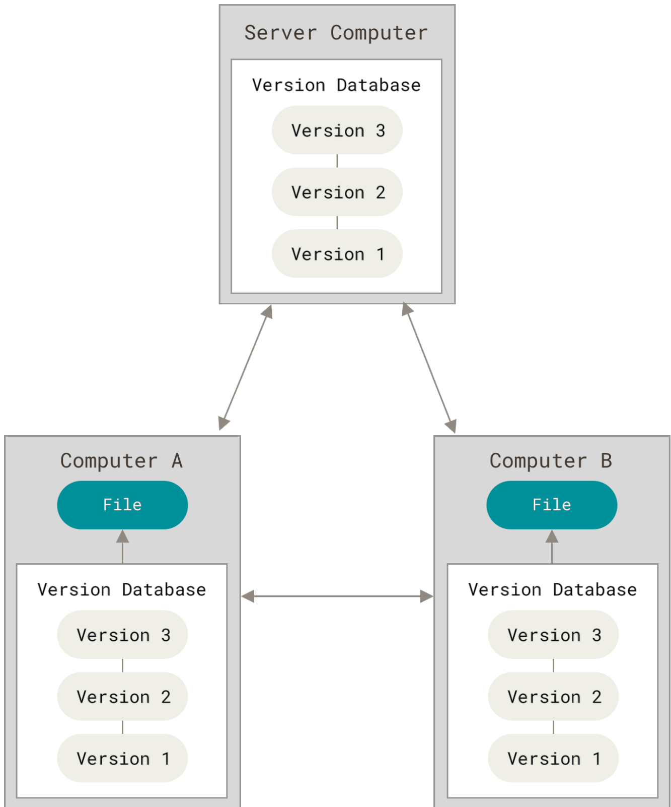
图表 3. 分布式版本控制.
