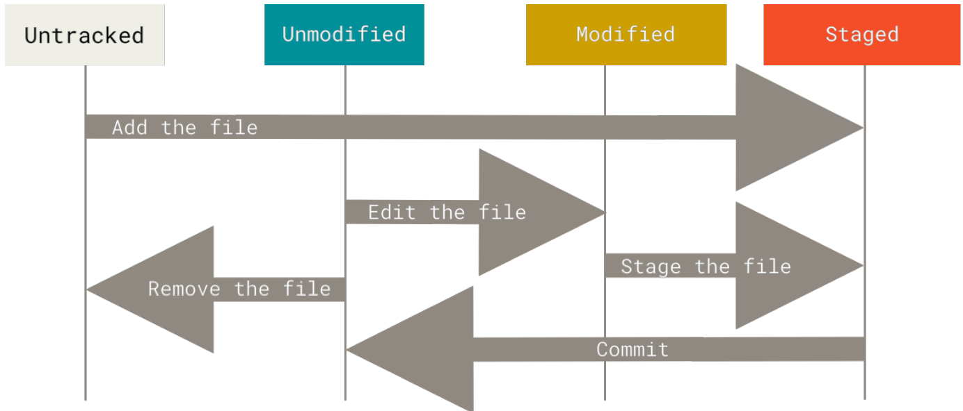
图表 8. 文件的状态变化周期
