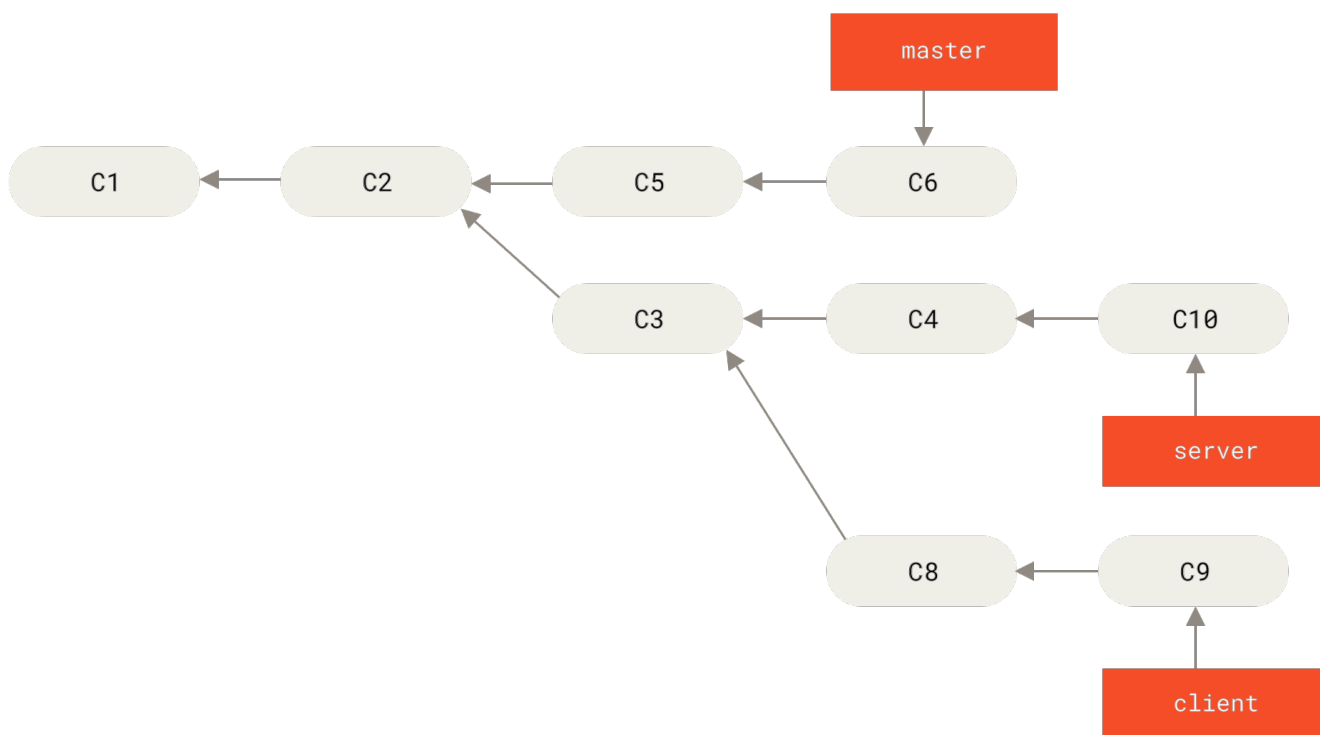
图表 39. 从一个主题分支里再分出一个主题分支的提交历史
