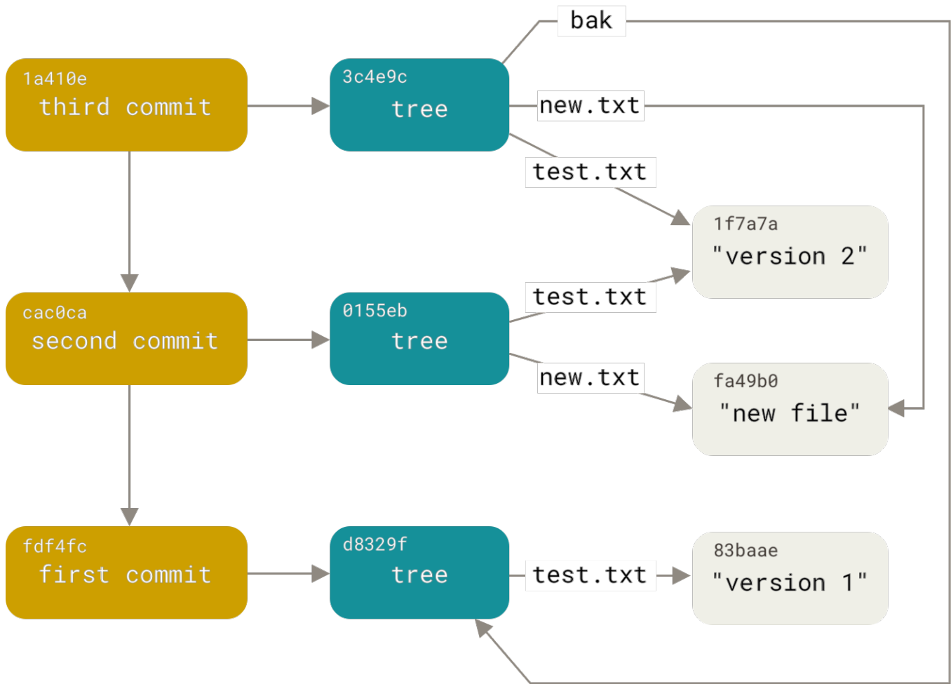
图表 150. 你的 Git 目录下所有可达的对象。
