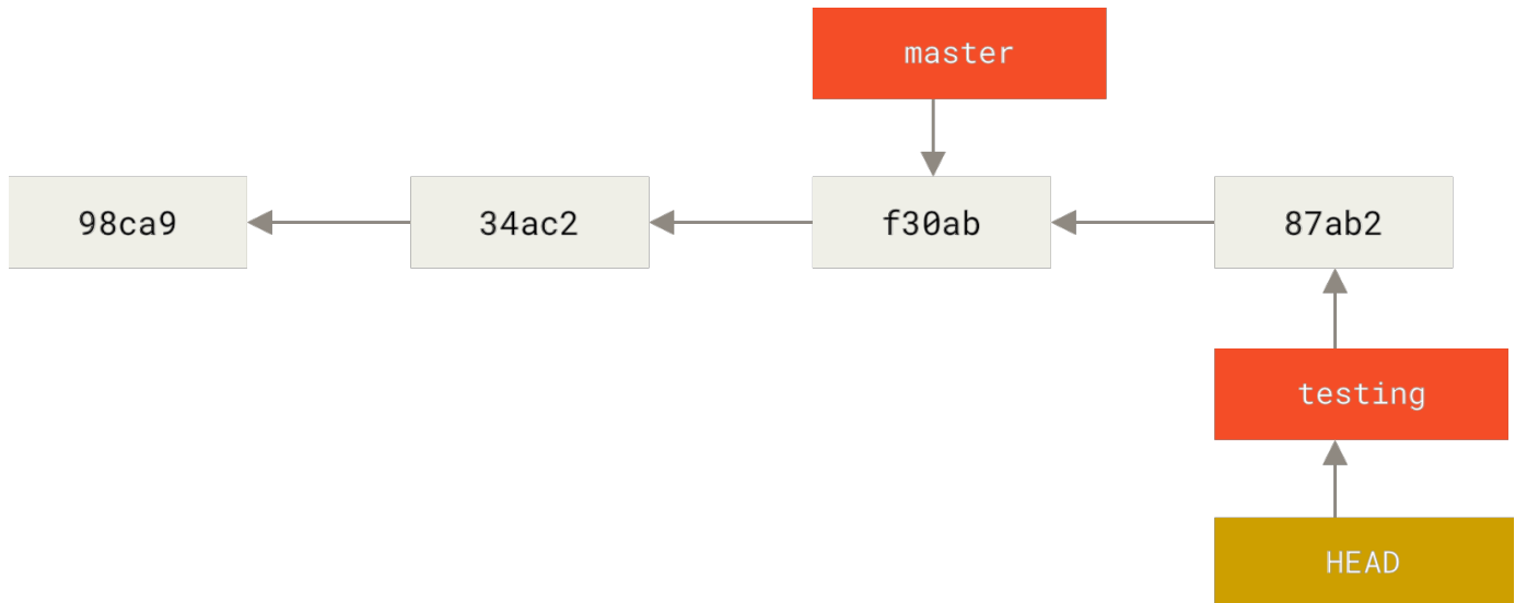
图表 15. HEAD 分支随着提交操作自动向前移动
