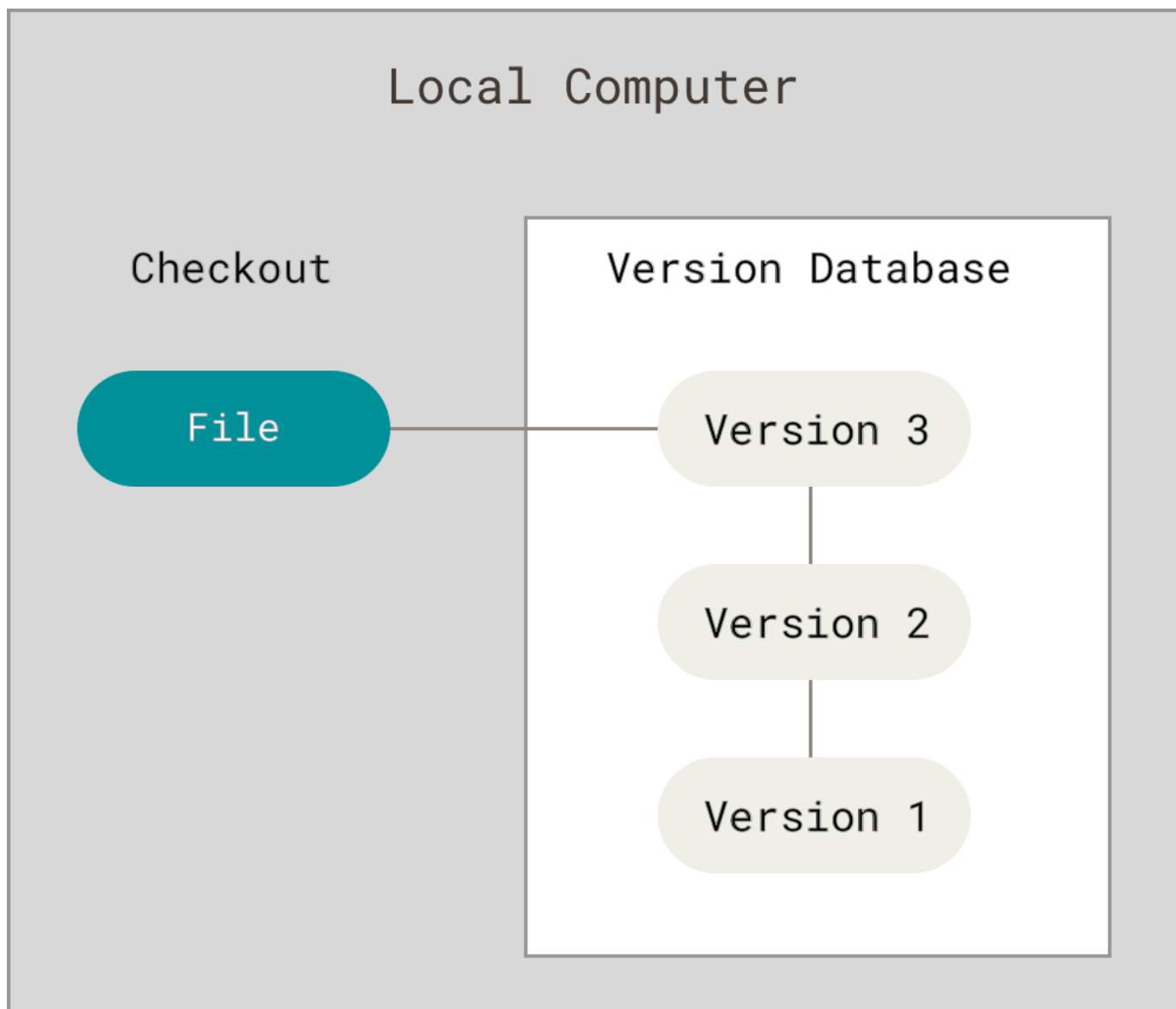
图表 1. 本地版本控制.
