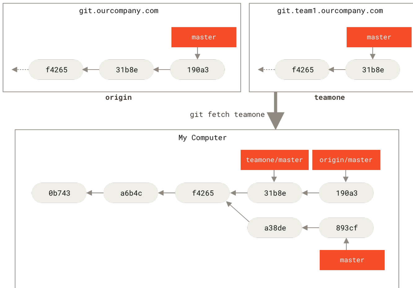
图表 34. 远程跟踪分支 teamone/master
