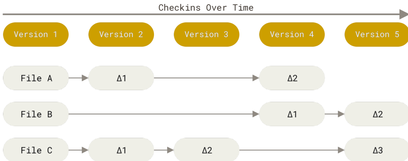
图表 4. 存储每个文件与初始版本的差异。
