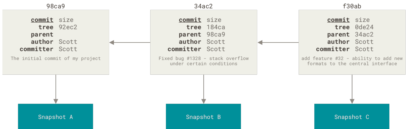
图表 10. 提交对象及其父对象
