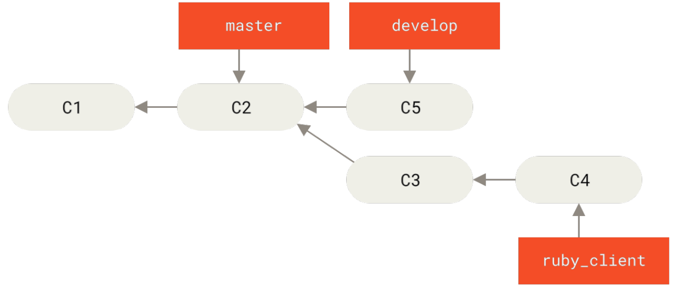
图表 75. 合并主题分支前。
