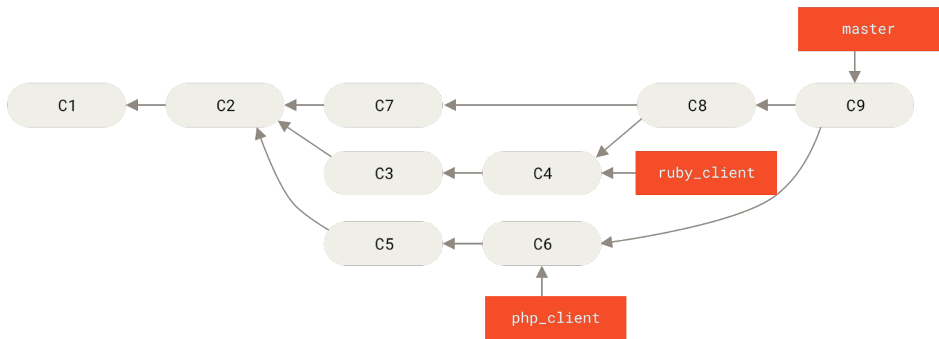
图表 74. 合并主题分支之后。
