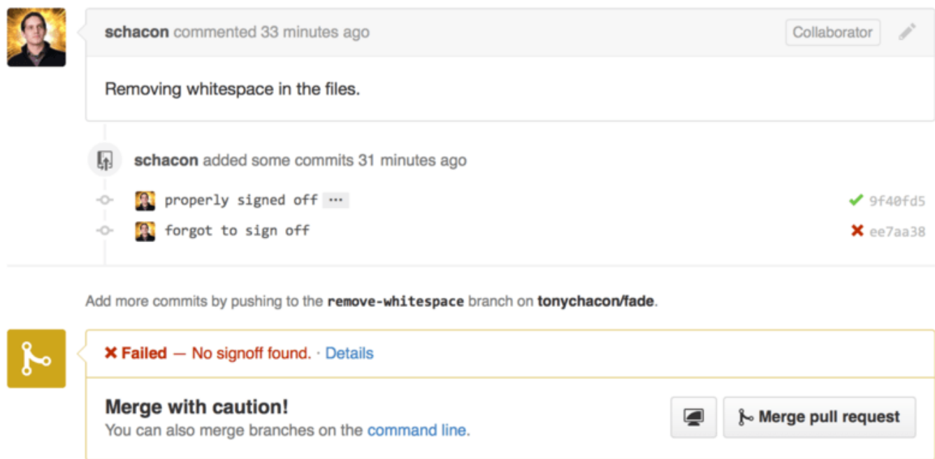
图表 136. 通过 API 的提交状态
