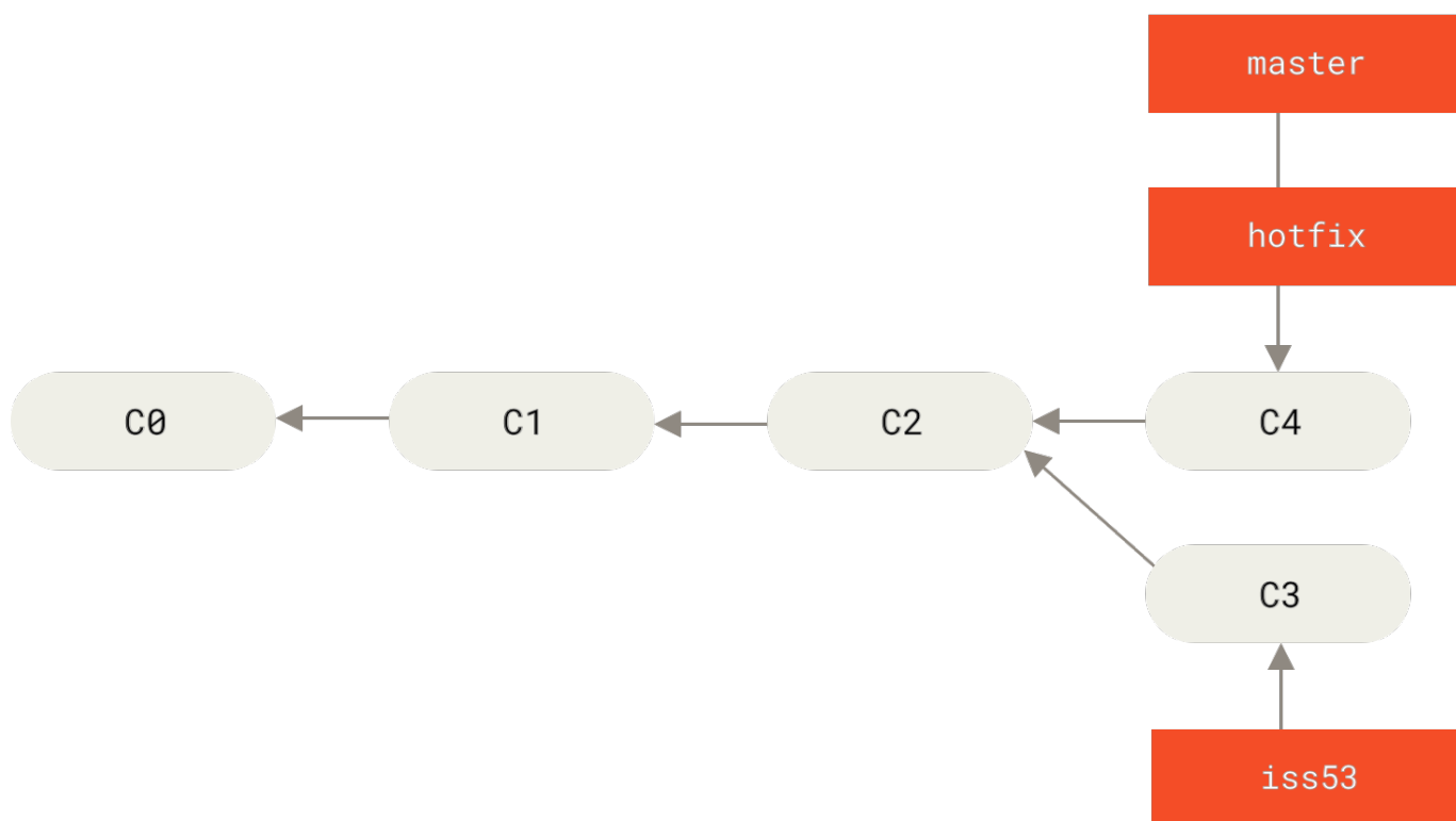
图表 22. master 被快进到 hotfix
