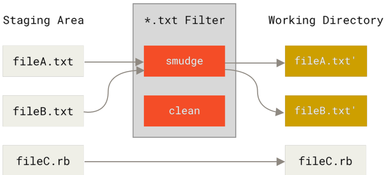
图表 144. “smudge” 过滤器会在文件被检出时触发
