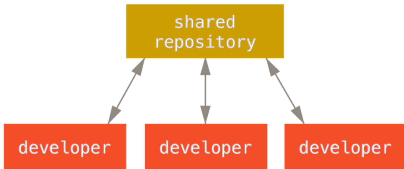
图表 54. 集中式工作流。
