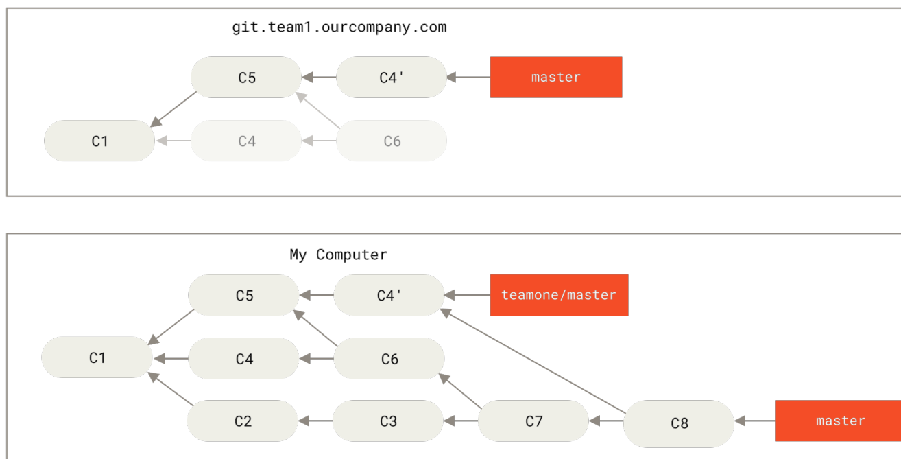
图表 47. 你将相同的内容又合并了一次，生成了一个新的提交
