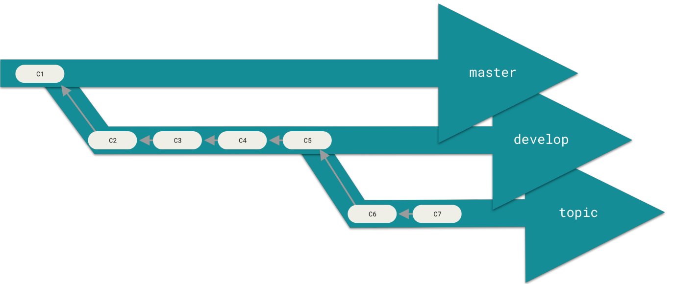
图表 27. 趋于稳定分支的流水线（“silo”）视图
