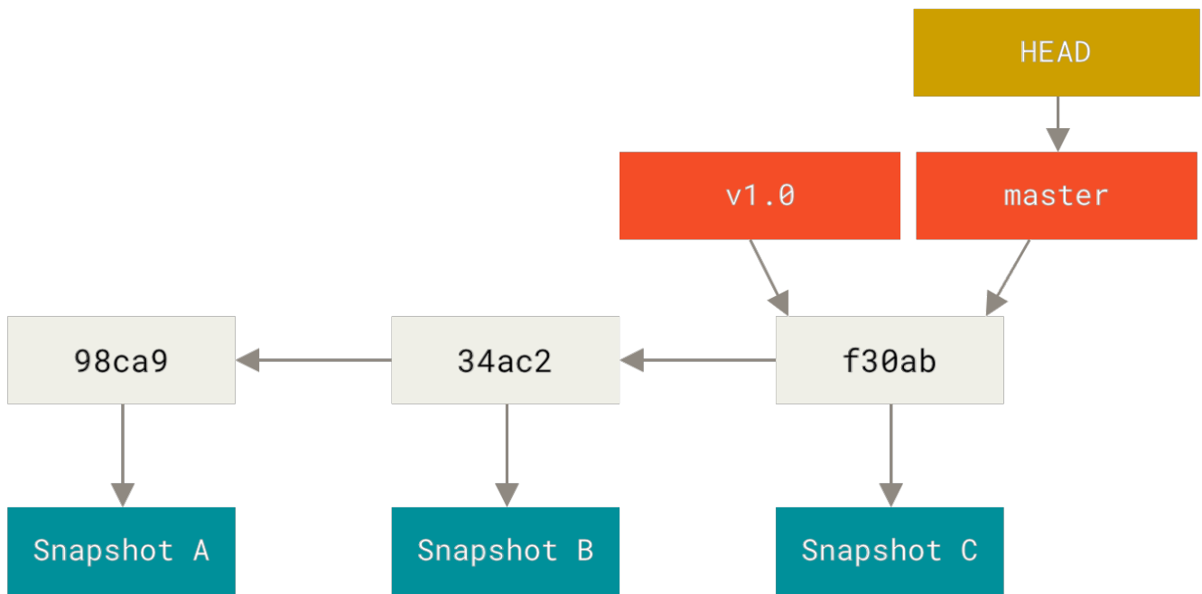
图表 11. 分支及其提交历史
