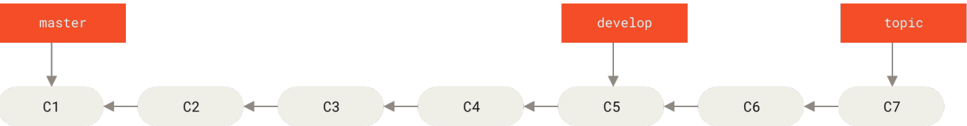
图表 26. 趋于稳定分支的线性图
