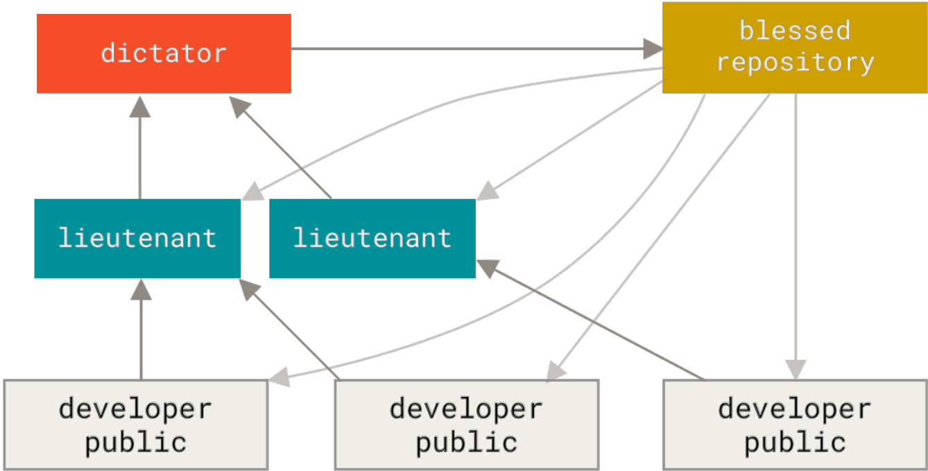
图表 56. 主管与副主管工作流。
