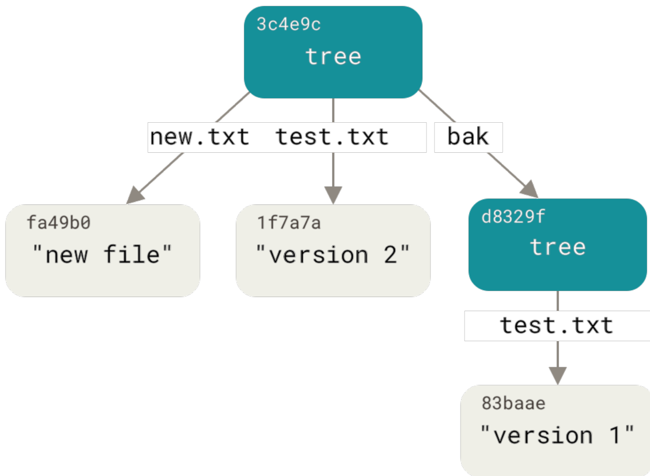
图表 149. 当前 Git 的数据内容结构。
