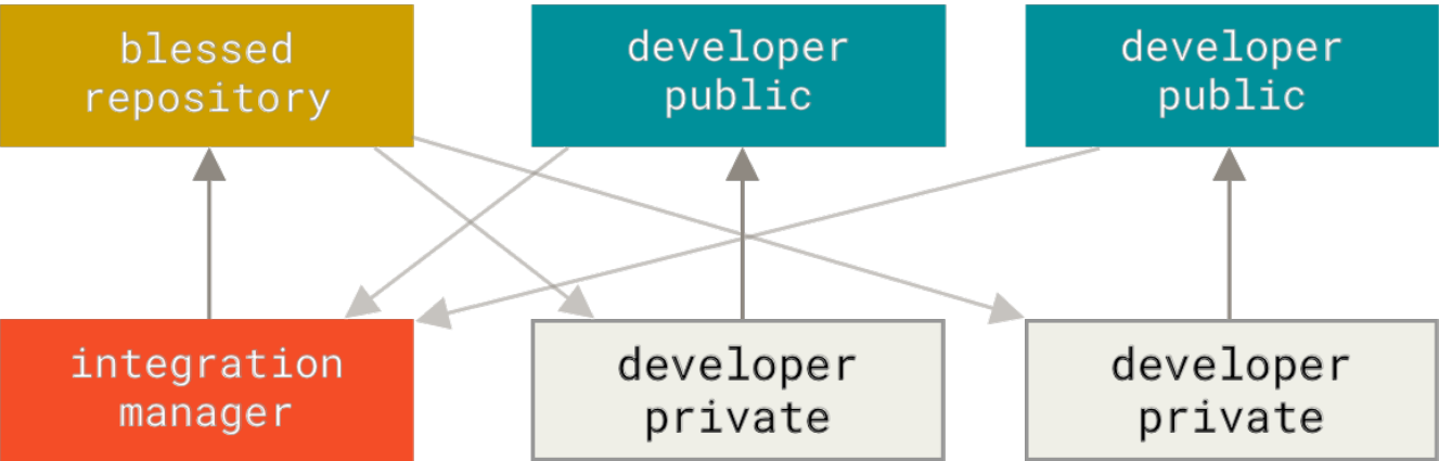
图表 55. 集成管理者 workflow。
