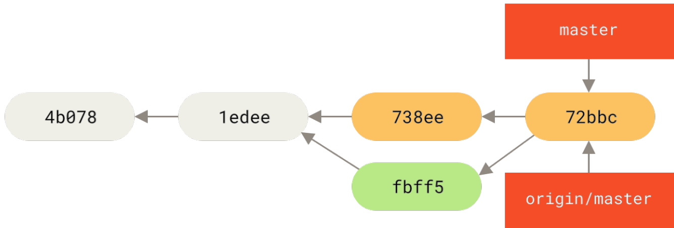
图表 60. 推送到 origin 服务器后 John 的历史
