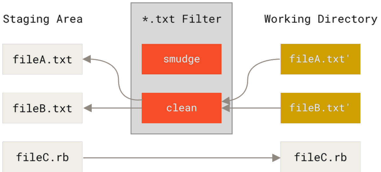
图表 145. “clean” 过滤器会在文件被暂存时触发
