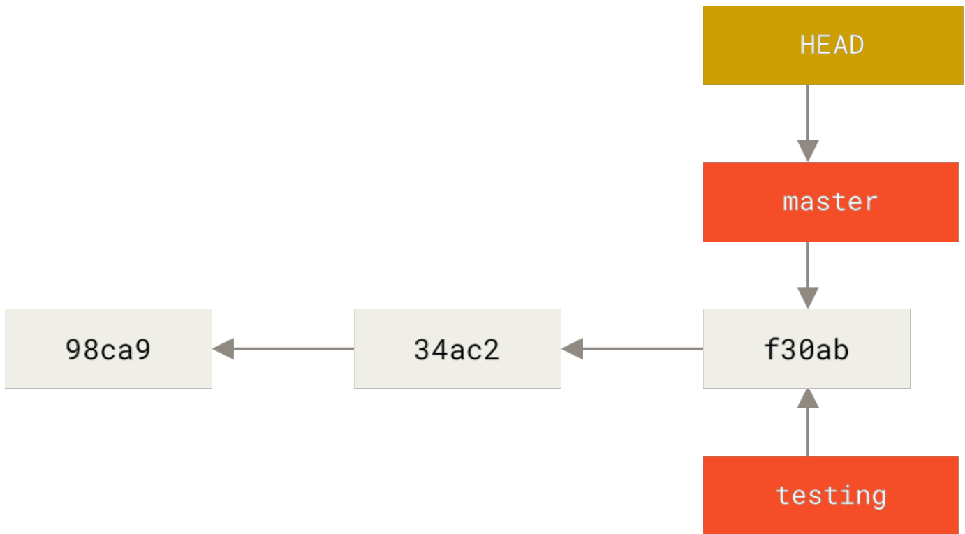
图表 13. HEAD 指向当前所在的分支
