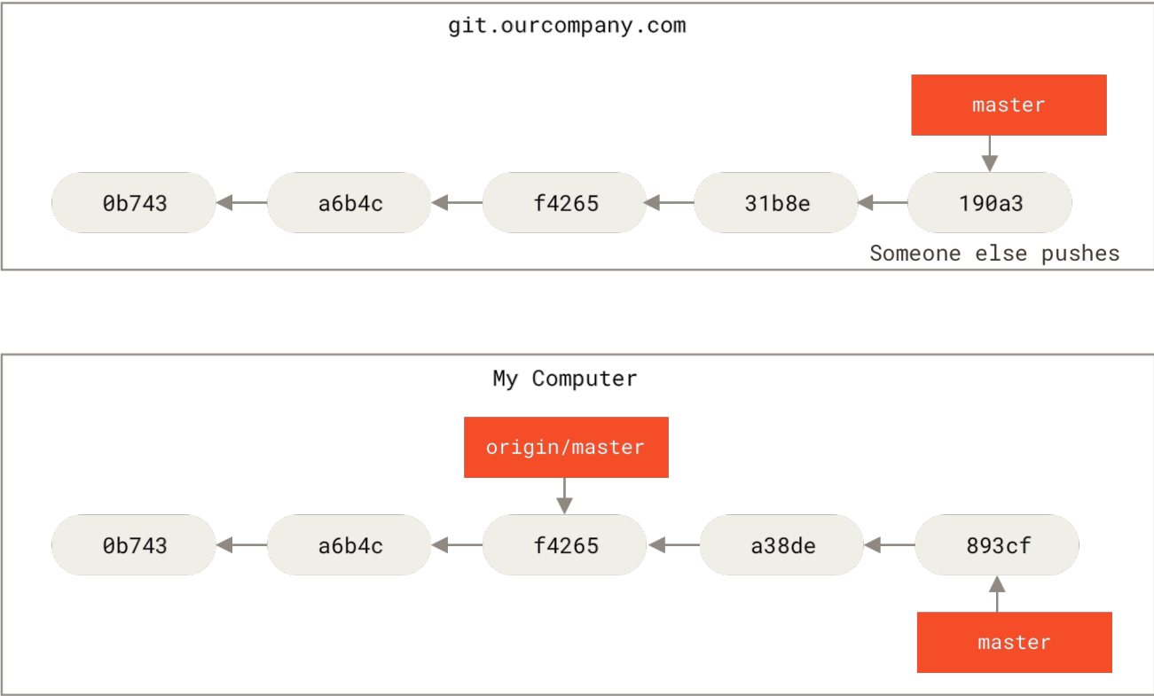
图表 31. 本地与远程的工作可以分叉
