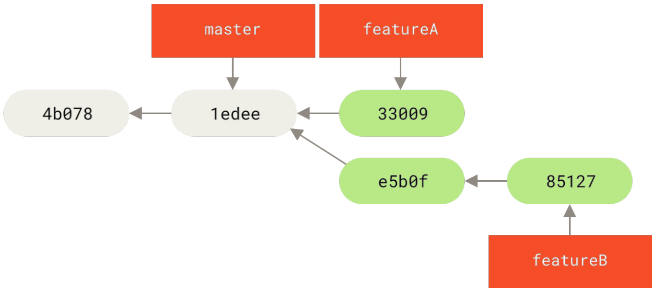
图表 66. Jessica 的初始提交历史
