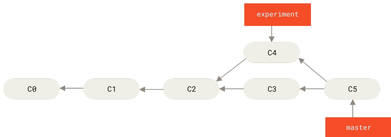
图表 36. 通过合并操作来整合分叉的历史
