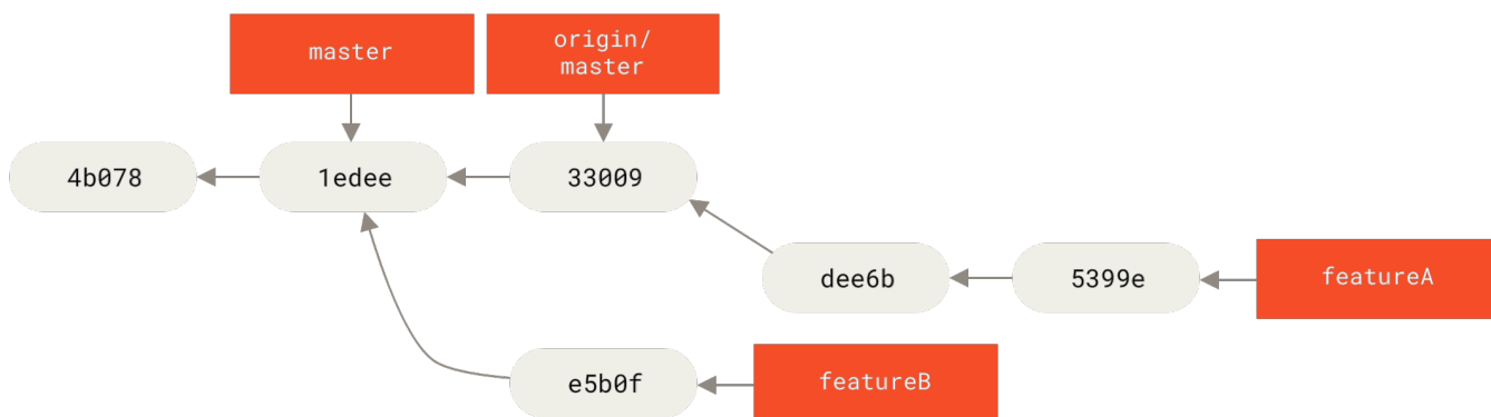
图表 71. featureA 工作之后的提交历史
