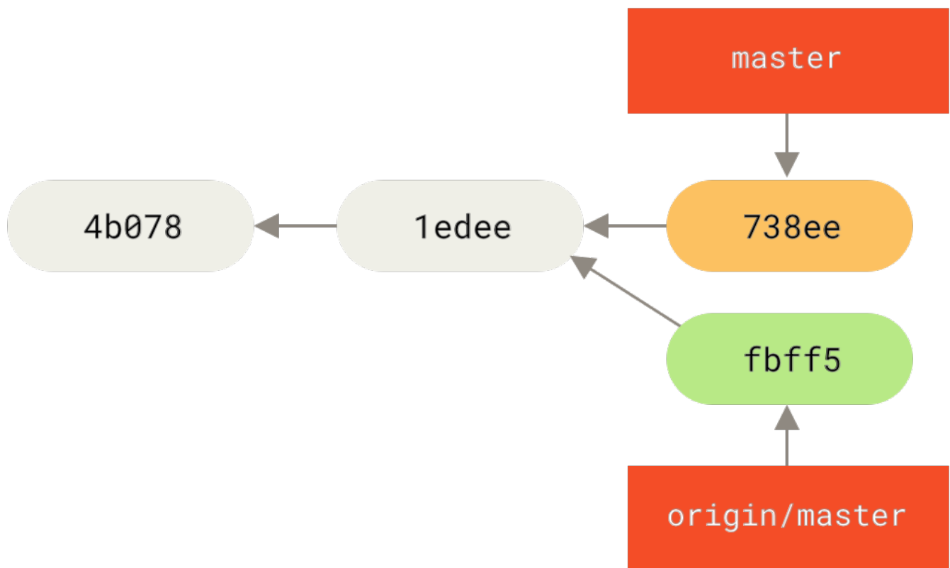
图表 58. John 的分叉历史
