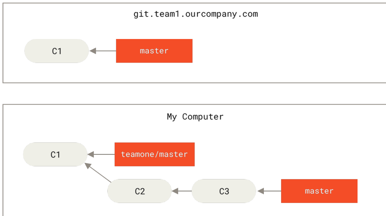
图表 44. 克隆一个仓库，然后在它的基础上进行了一些开发
