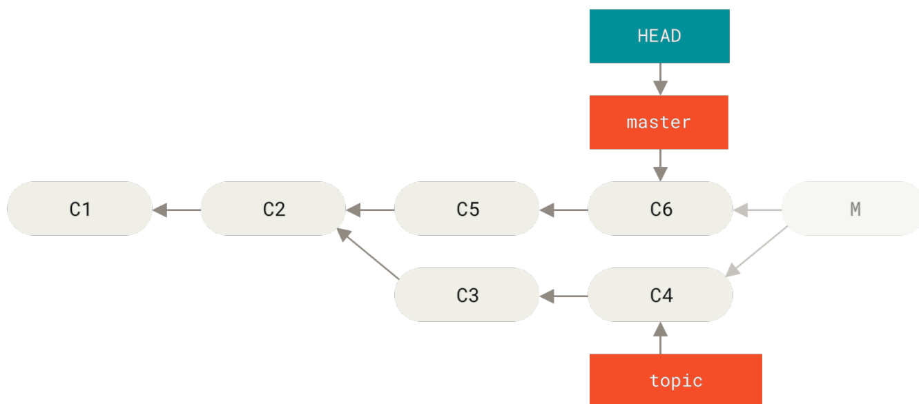
图表 139. 在 git reset --hard HEAD~ 之后的历史
