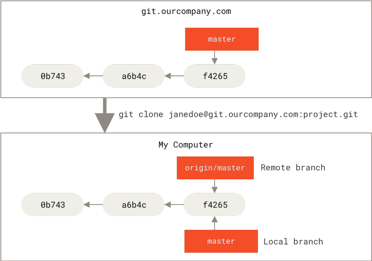
图表 30. 克隆之后的服务器与本地仓库
