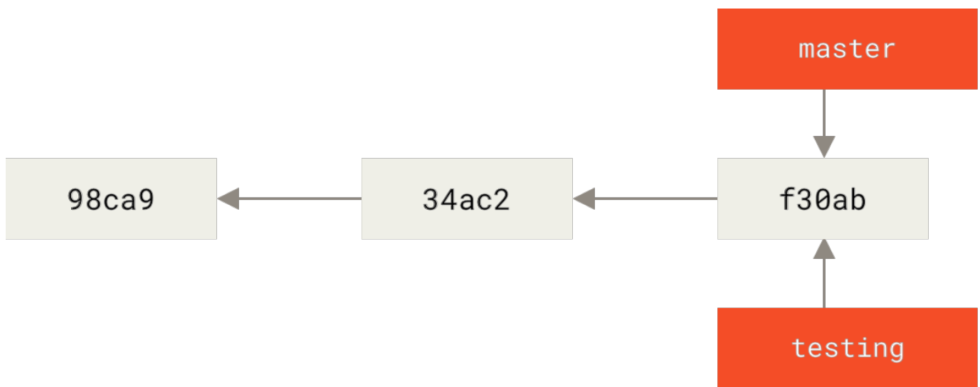
图表 12. 两个指向相同提交历史的分支
