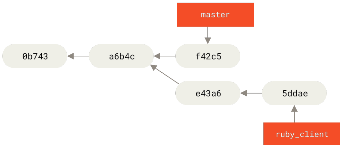
图表 80. 拣选之前的示例历史。
