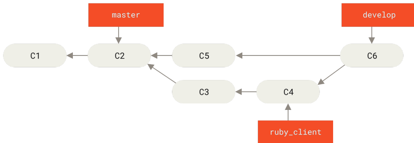
图表 76. 合并主题分支后。
