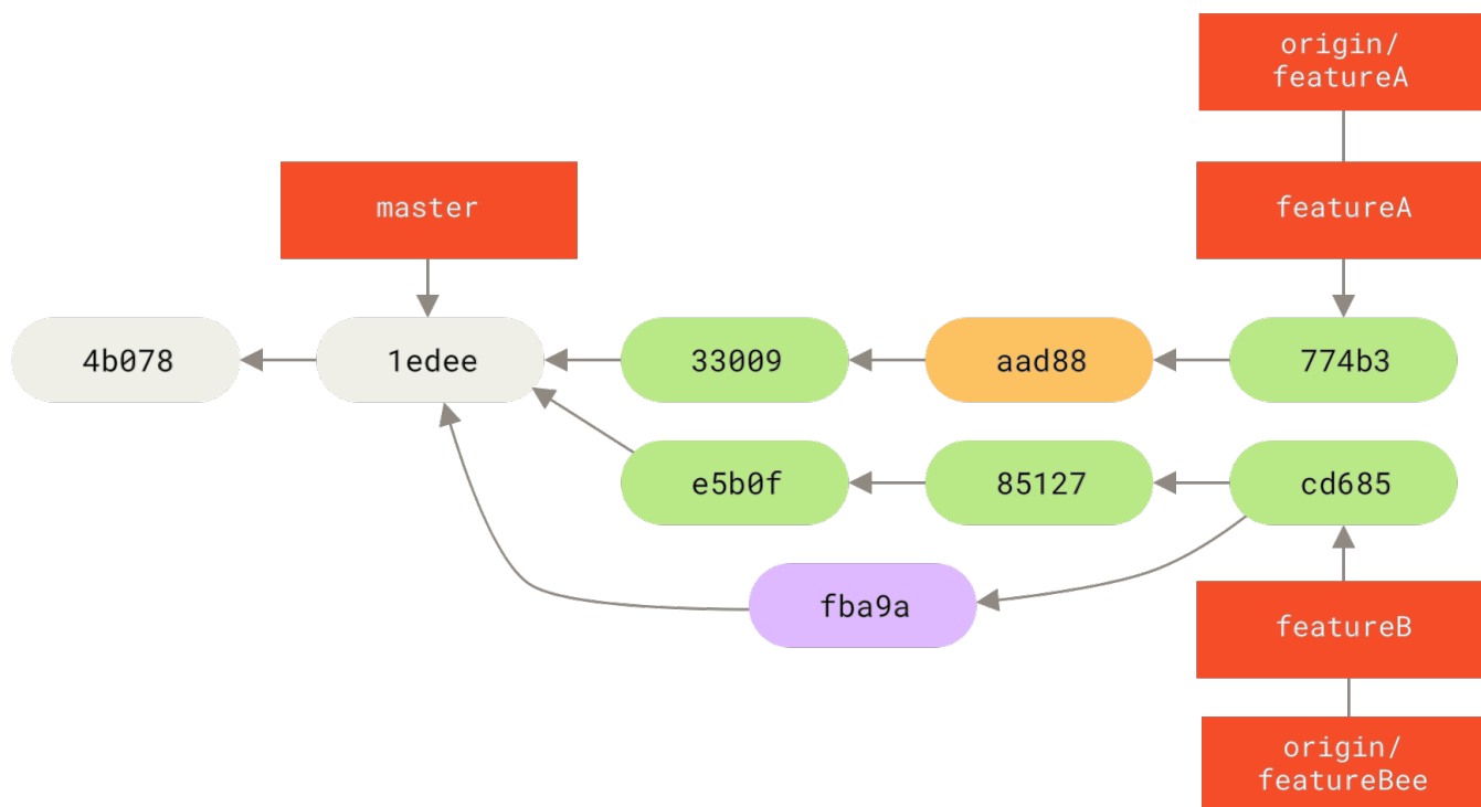
图表 67. 在一个主题分支提交后 Jessica 的历史
