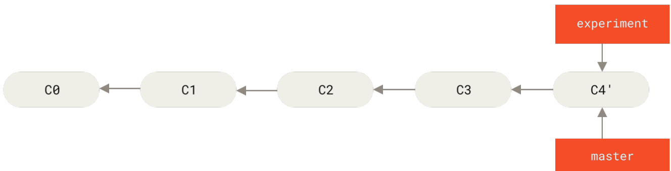
图表 38. master 分支的快进合并
