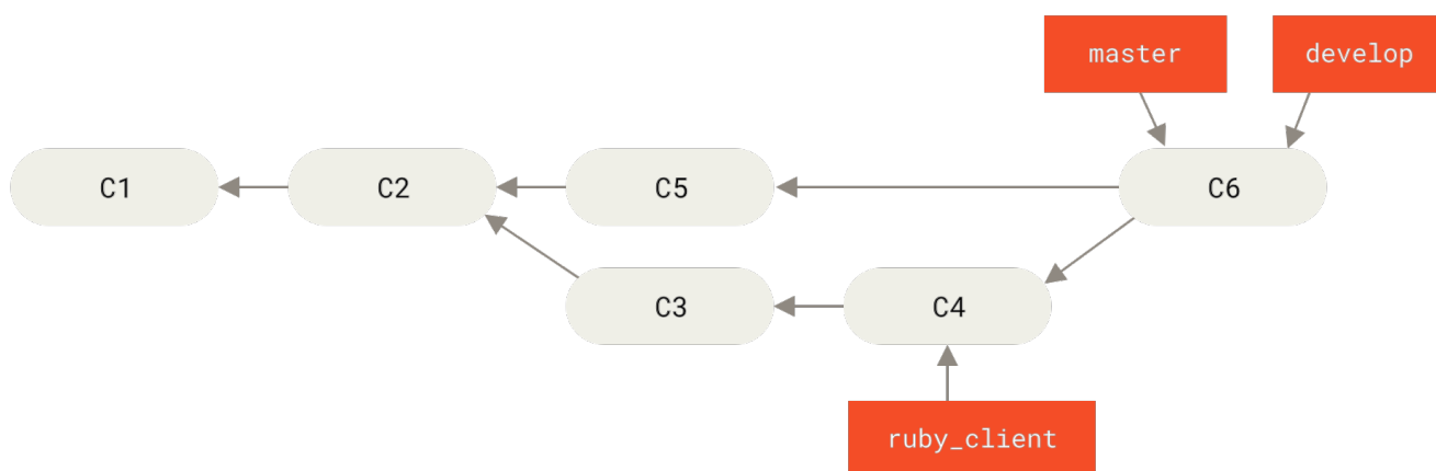
图表 77. 一次发布之后。
