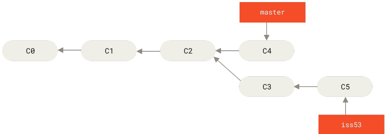
图表 23. 继续在 iss53 分支上的工作
