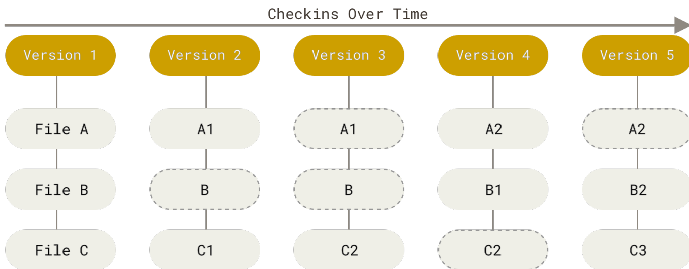
图表 5. 存储项目随时间改变的快照。
