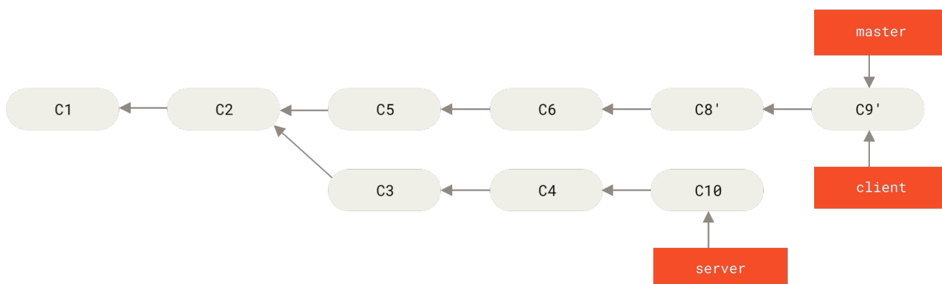
图表 41. 快进合并 master 分支，使之包含来自 client 分支的修改
