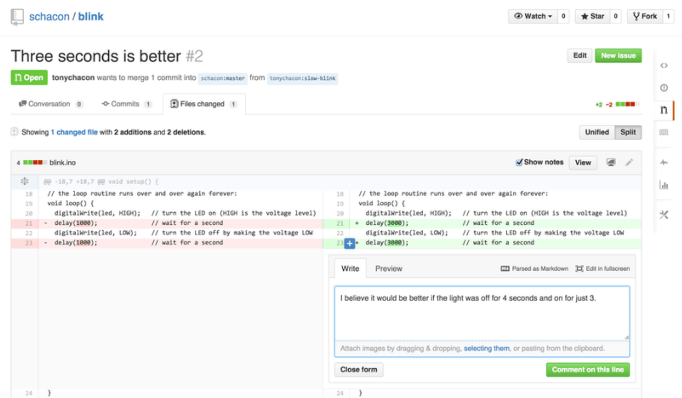
图表 93. 对拉取请求内的特定一行发表评论
