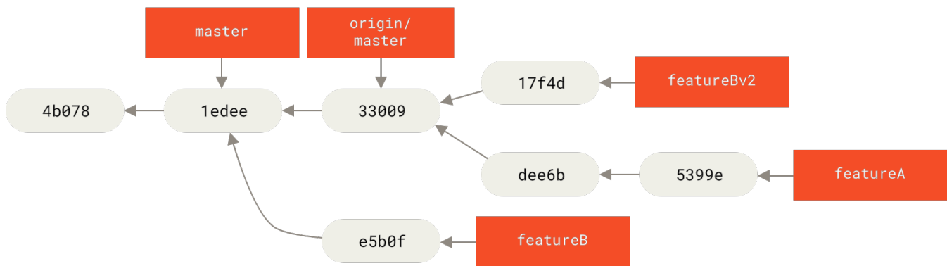
图表 72. featureBv2 工作之后的提交历史
