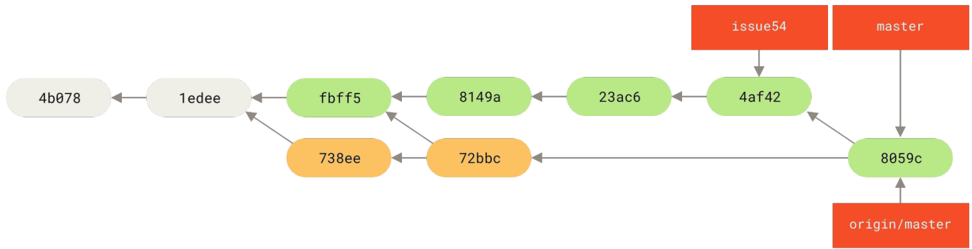
图表 64. 推送所有的改动回服务器后 Jessica 的历史
