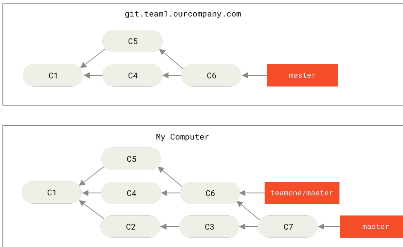
图表 45. 抓取别人的提交，合并到自己的开发分支
